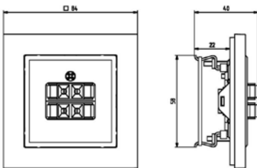
Art. no: 62 210 27
