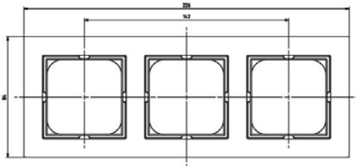
Art. no: 18 944 26/18 944 32
