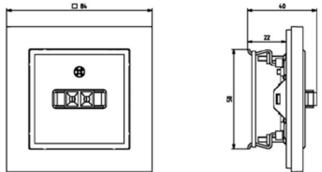
Art. no: 62 210 26
