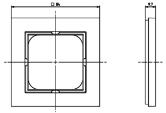
Art. no: 18 944 30
