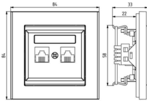
Art. no: 51 188 32
