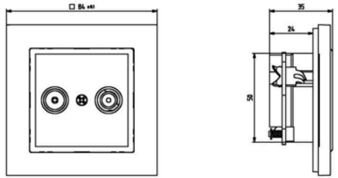
Art. no: 60 700 56/60 700 57
