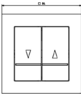
Art. no: 18 944 14
