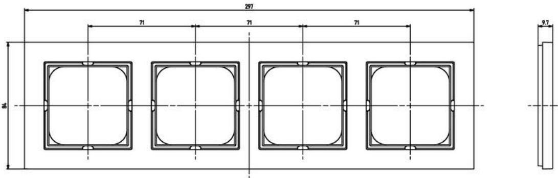
Art. no: 18 944 27
