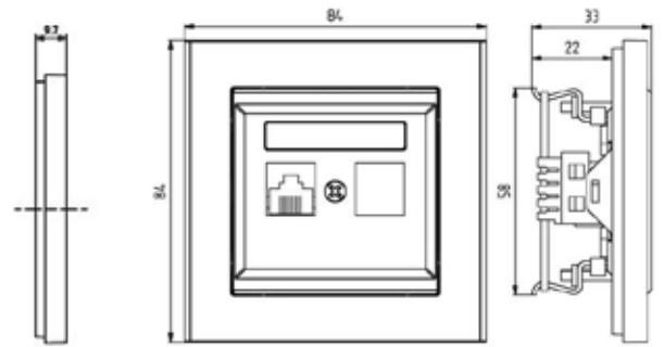
Art. no: 51 188 31
