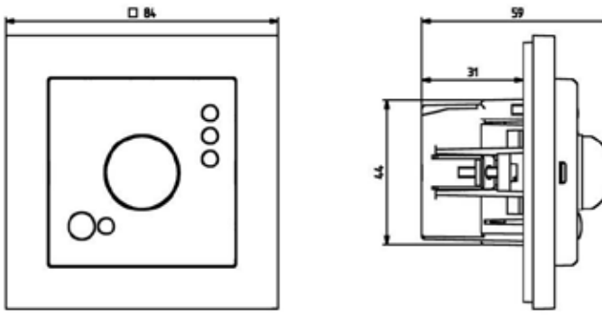
Art. no: 130 00 00
