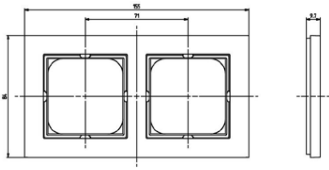
Art. no: 18 944 25/18 944 31
