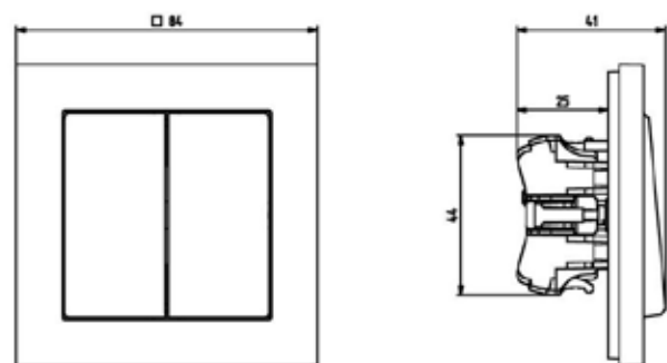
Art. no: 18 944 05/18 944 06/ 18 944 10
