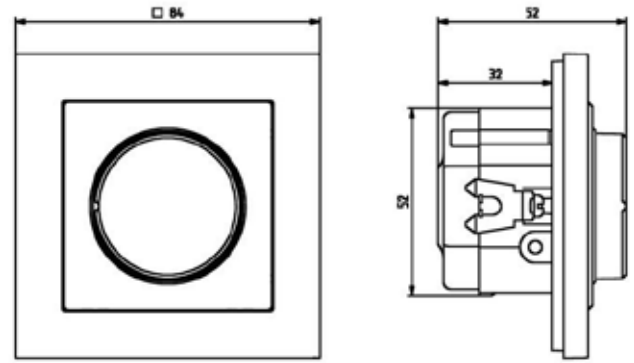
Art. no: 13 772 01/13 772 02
