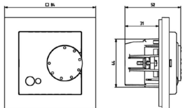
Art. no: 85 800 75
