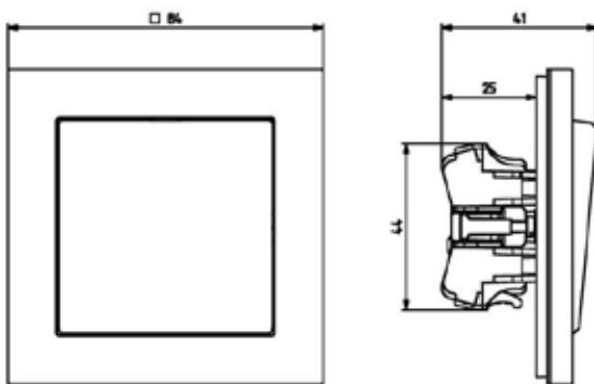
Art. no: 18 944 00/18 944 07/ 18 944 08/18 944 11
