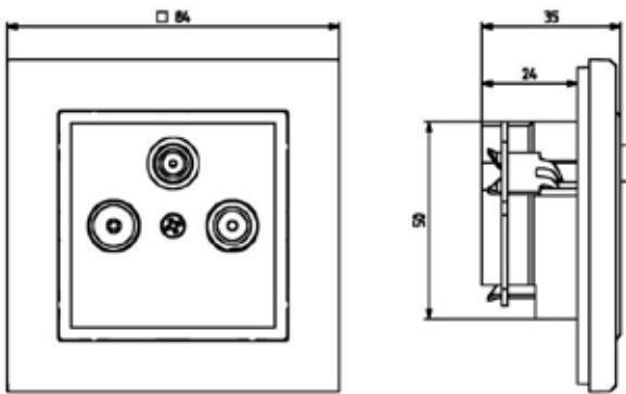
Art. no: 60 700 58/60 700 59
