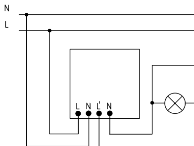
Kopplingsschema/Kytentäkaavio/Wiring diagram
