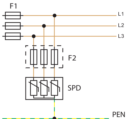
TN-C
