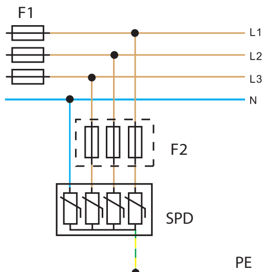
TN-S
